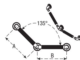
Grab Bar 135°
