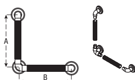
Grab Bar 90°
